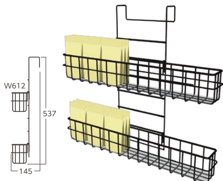
28 薄型金型2段什器 ■材質/スチール
