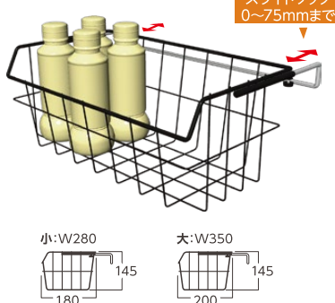
29 ワ이어エクステンダー黒 ■材質/スチール、樹脂 既製品
