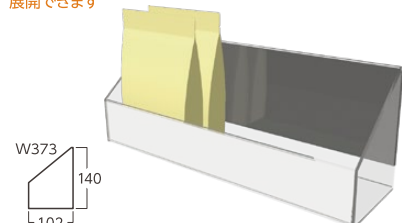
33 マグネット什器 ■材質/樹脂、マグネット
